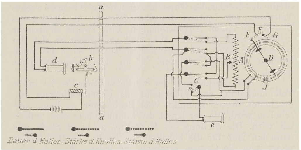
Abbildung 3: Bauanleitung des Akustometers von Exner, in: Sigmund Exner, Über die Akustik von Hörsälen und ein Instrument, sie zu bestimmen . Wien, Selbstverlag 1905.
