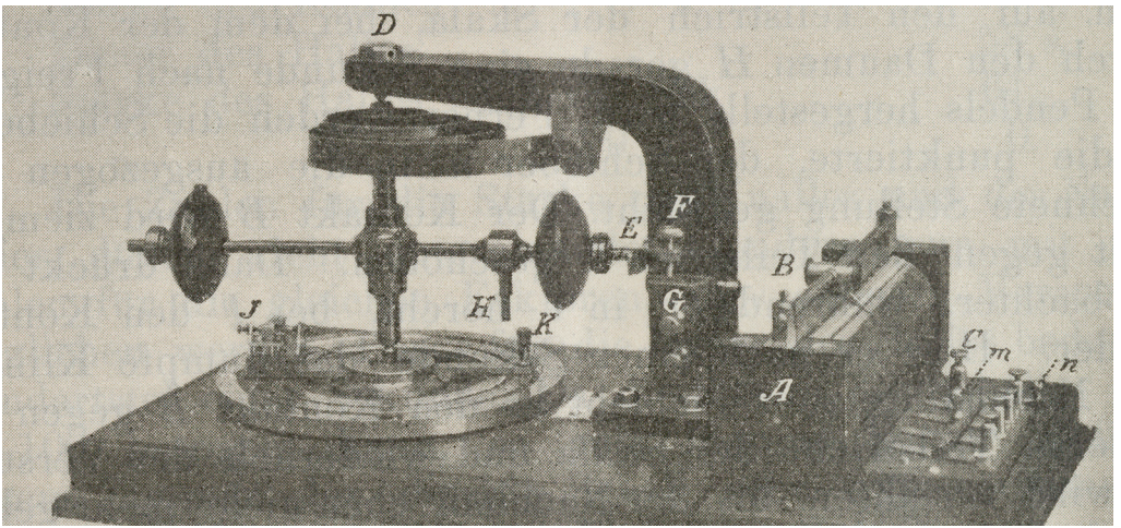
Abbildung 2: Fotografie des Akustometers von Exner, in: Sigmund Exner, Über die Akustik von Hörsälen und ein Instrument, sie zu bestimmen . Wien, Selbstverlag 1905.
